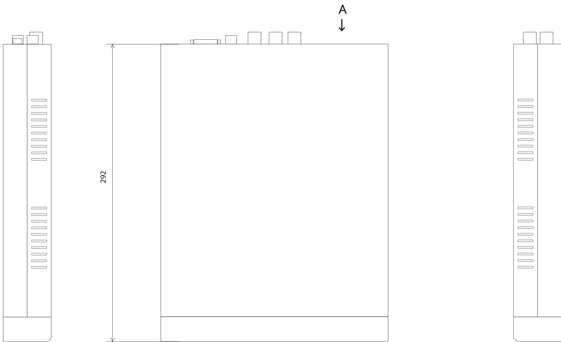
A 矢視図
