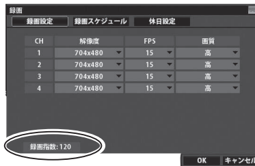
▼DVR-S220の録画設定画面
