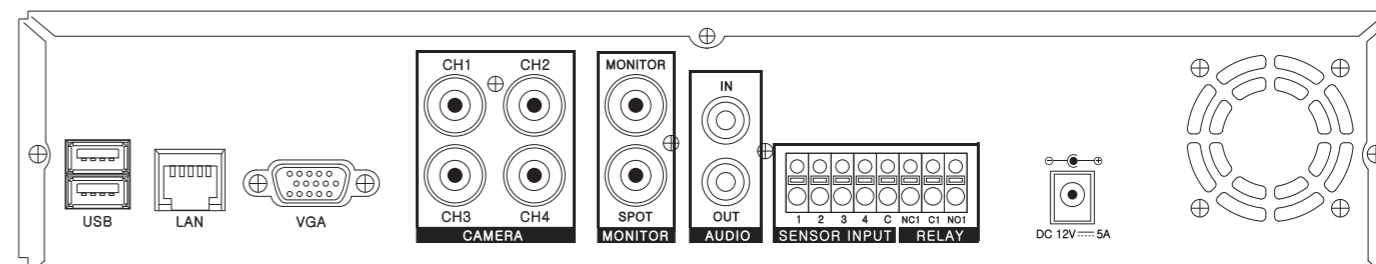
A 矢視図
